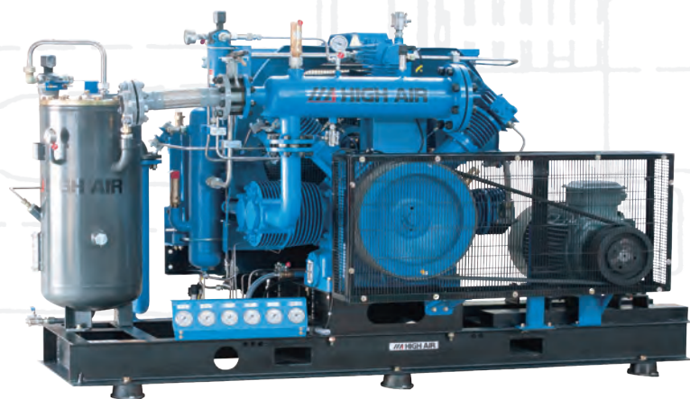
HEM系列 流量：10-25Nm 3 /hr 压力：150-250Bar
